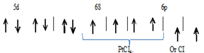
Рисунок 1. Схема образования иона PtCl_6^{2-}
